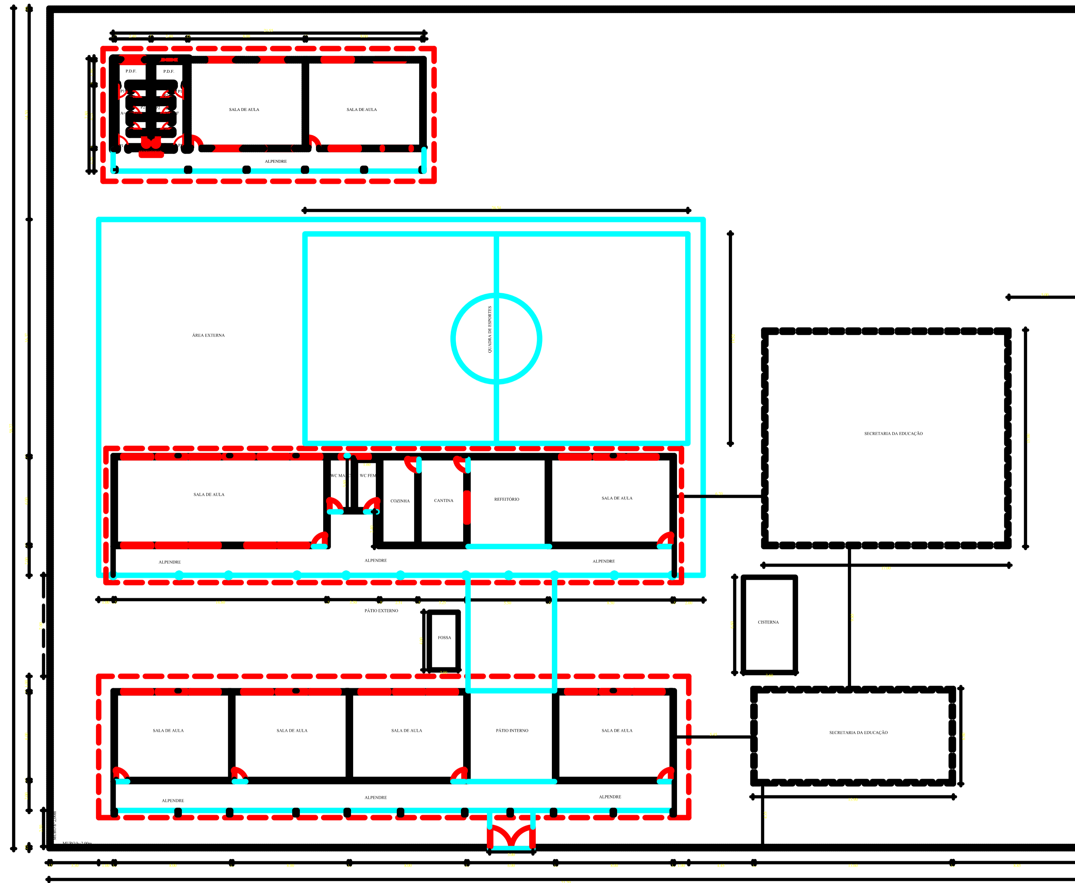
1 PLANTA BAIXA ESCALA: 1:200 LEGENDA: ■ PAREDE EXISTENTE ■ PAREDE PROJETADA ■ PAREDE A DEMOLIR
