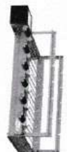
Itagrill 6 Espetos Altura: 28,5 cm Profundidade: 65,0 cm Frente: 71,5 cm Frente com Motor: 82,0 cm Código: 9121
