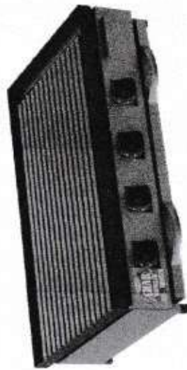
Char Broiler 850x500 Altura: 22,0 cm Profundidade: 57,0 cm Frente: 85,0 cm Código: 11036
