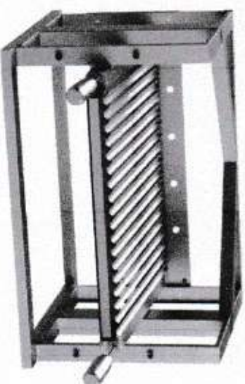
Elevante 5 Espetos Altura: 43,5 cm Profundidade: 50,0 cm Frente: 71,5 cm Código: 9387
