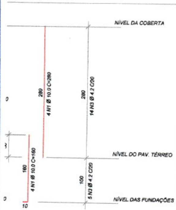
Detalhe dos Pilares ALA 1:50
